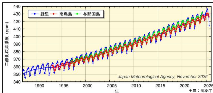
図 1.1 二酸化炭素濃度の経年変化
