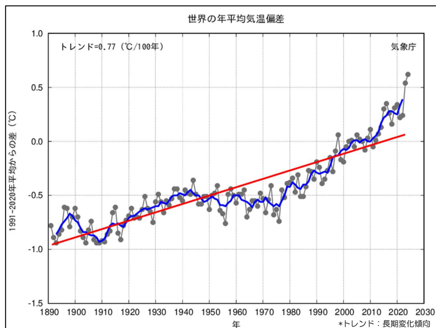
図 1.2 世界の年平均気温偏差
