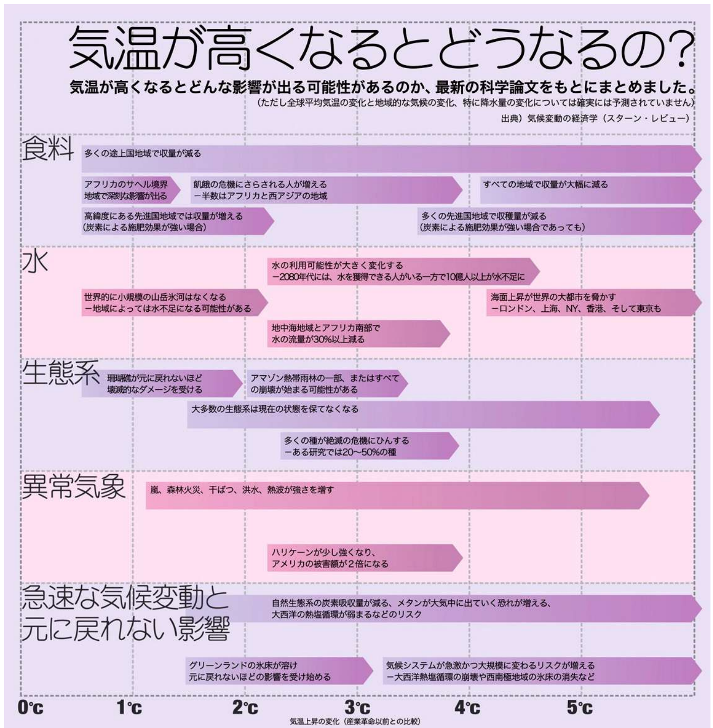
図 1.8 地球温暖化によるさまざまな影響
