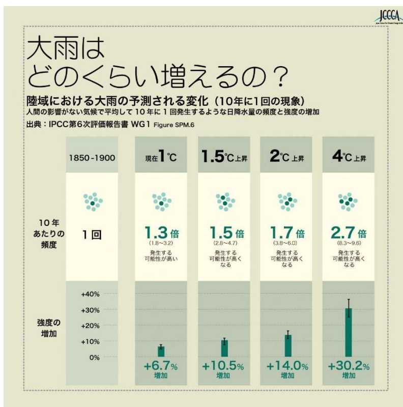
図 1.10 大雨の将来予測
