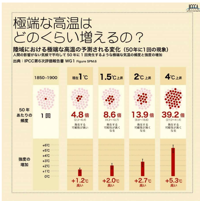
図 1.9 極端な高温の将来予測
