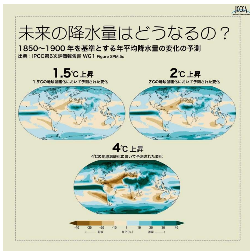
図 1.12 年平均降水量の将来予測（基準：1850～1900 年）
