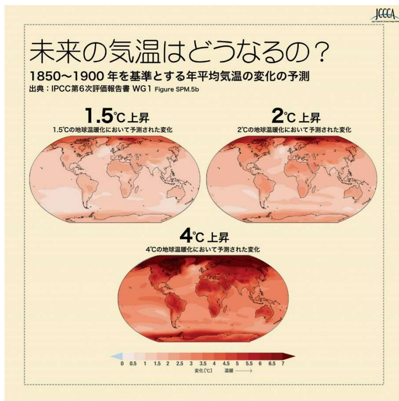
図 1.11 年平均気温の将来予測（基準：1850～1900 年）
