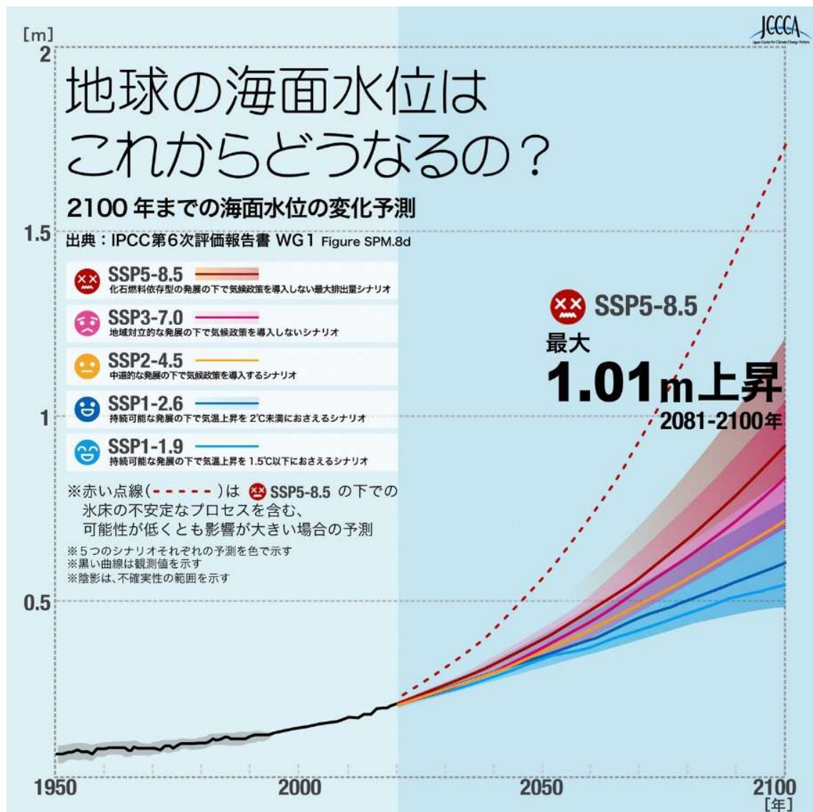
図 1.14 海面水位の将来予測
