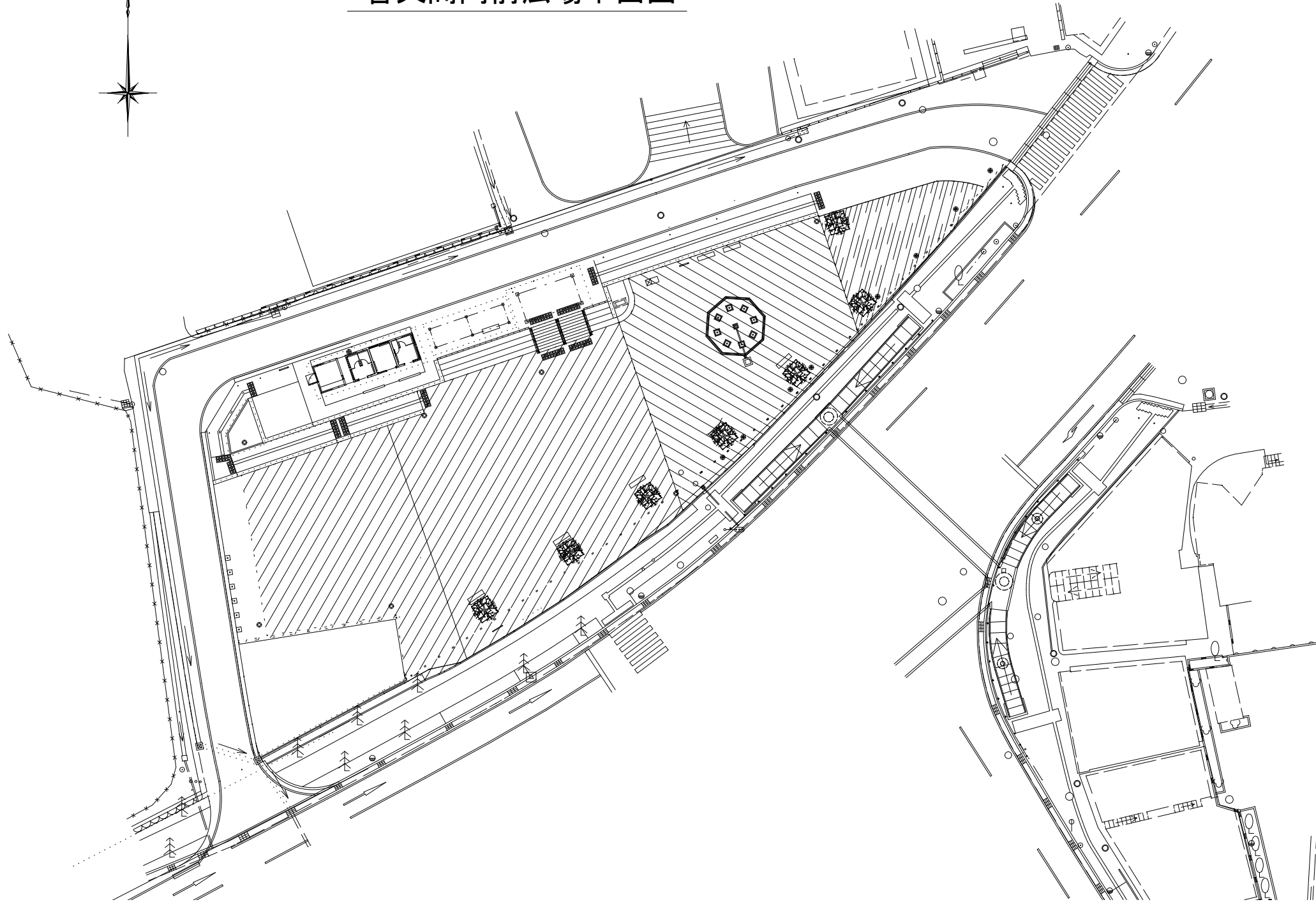
普天間門前広場平面図
