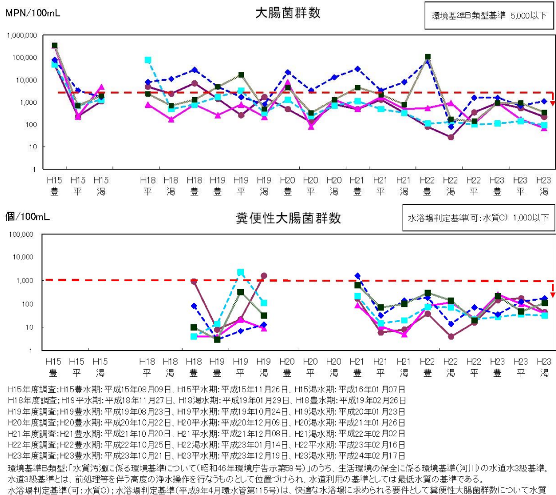
図 2-10 環境基準との比較 (生活環境項目 2/2)
