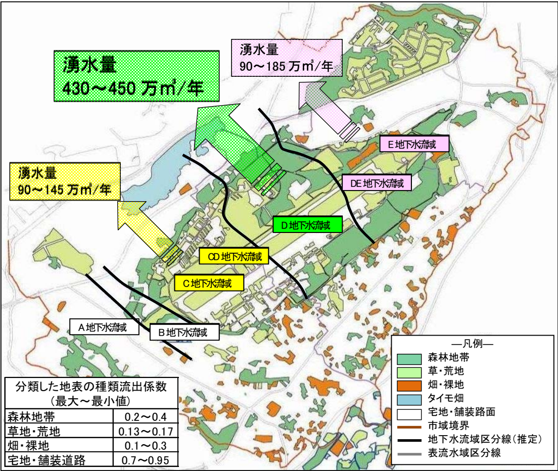
図- 4 普天間飛行場の水収支算定結果
