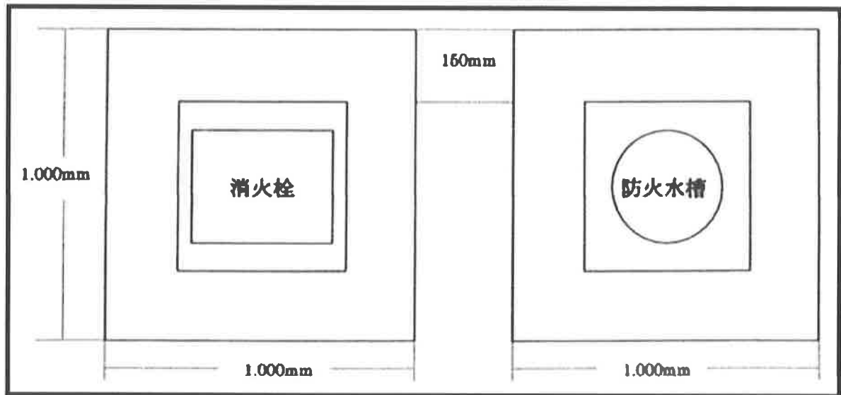
断面図
