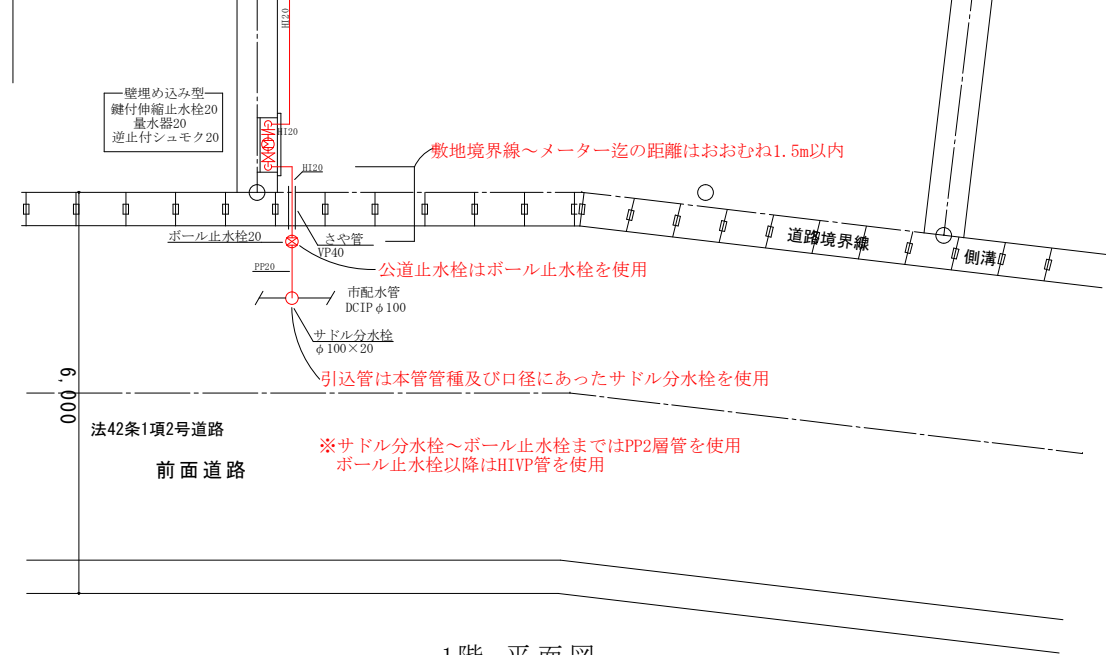
1階 平面図
