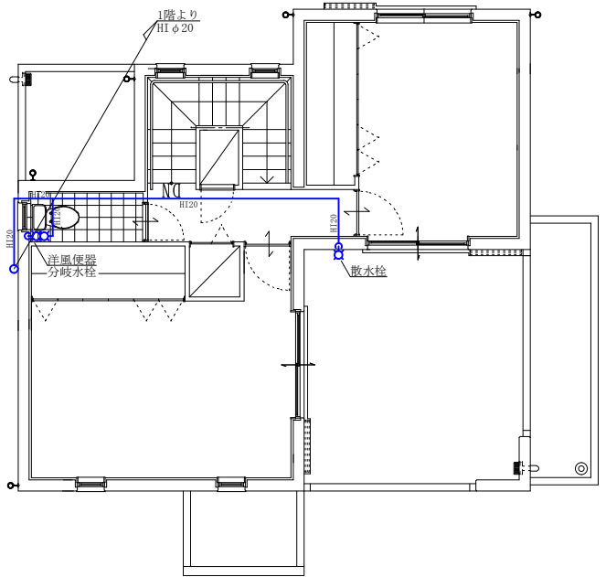
2階 平面図
