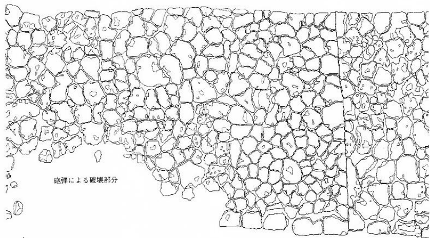
中城村北上原の石畳実測図（部分）
