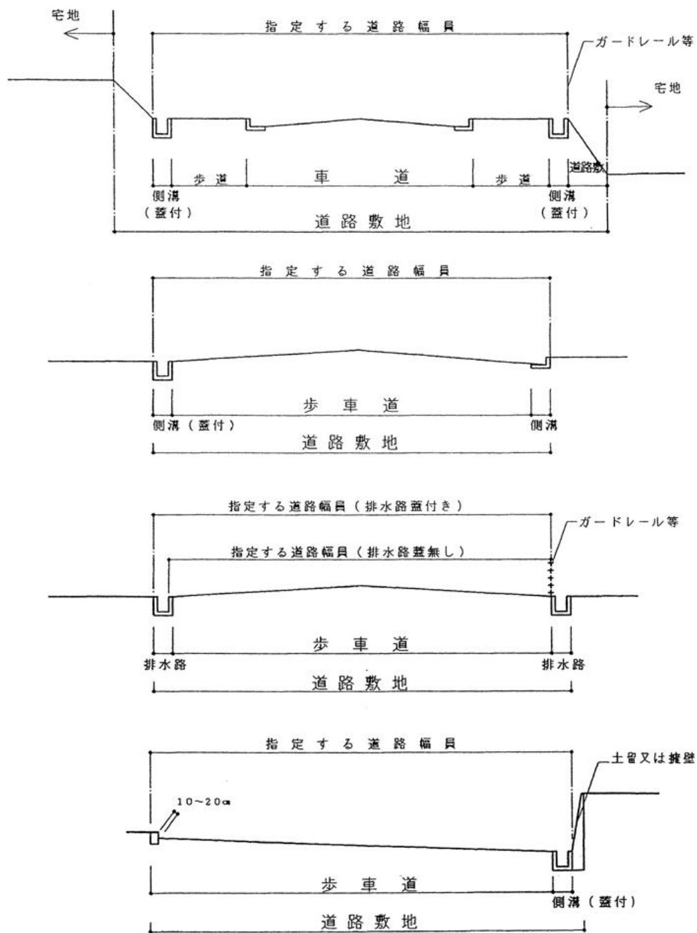
(図-4) 道路幅員の計測法
