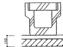
ESD落蓋側溝A型 A250以上とする
